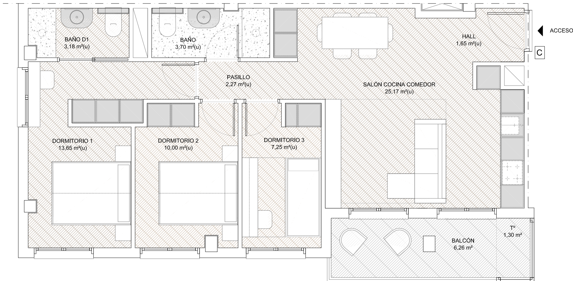
VIVIENDA P.1 - p.Baja - C
