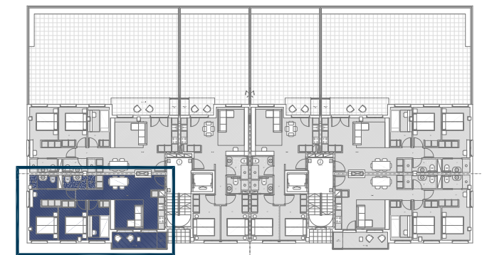
VIVIENDA PORTAL 1 Planta Baja Letra "C"
