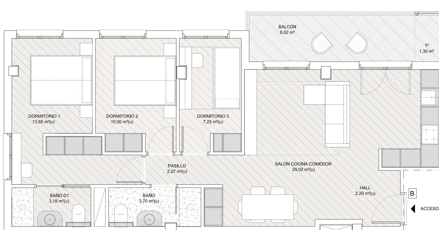
VIVIENDA P.1 - p.1 a - B
