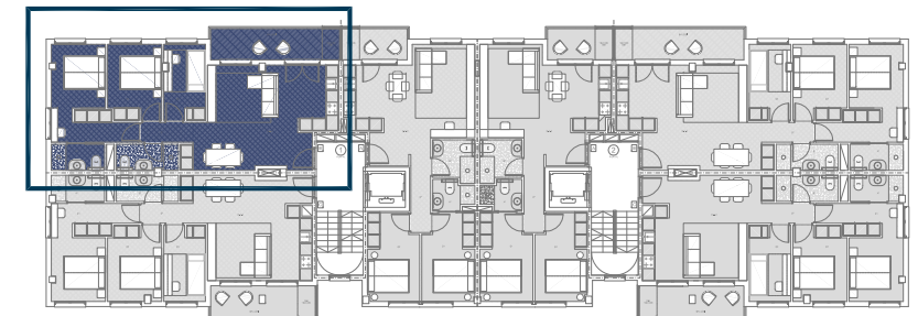
VIVIENDA PORTAL 1 Planta 1 a Letra "B"
