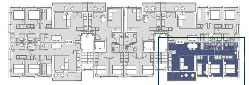
VIVIENDA PORTAL 2 Planta 1 a Letra "C"
